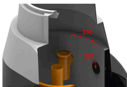
Рис.4 Септик «Загородный»
