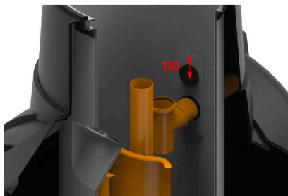
Рис.5 Септик «Коттеджный»
